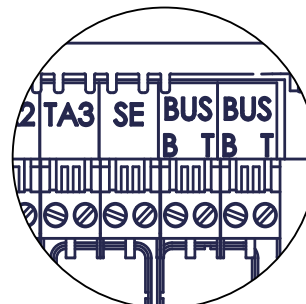
A vezérlőegység BUS sorkapcsa
