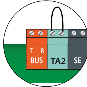
A kazán Bus sorkapcsa
