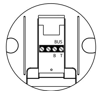
A távirányító sorkapcsa
