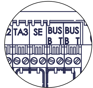
A vezérlőegység BUS sorkapcsa
